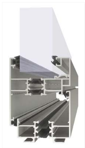
Ouverture extérieure
